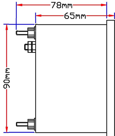
Yandan Görünüş / Side View
