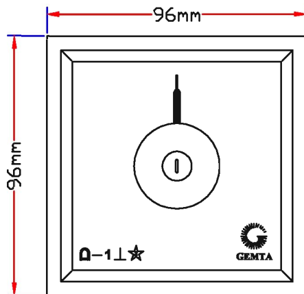
Önden Görünüş / Front View
