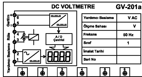
GV-201a BAĞLANTI ETİKETİ
