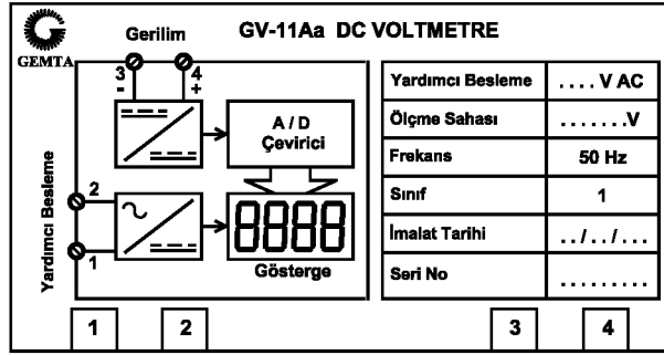
GV-11Aa BAĞLANTI ETİKETİ
