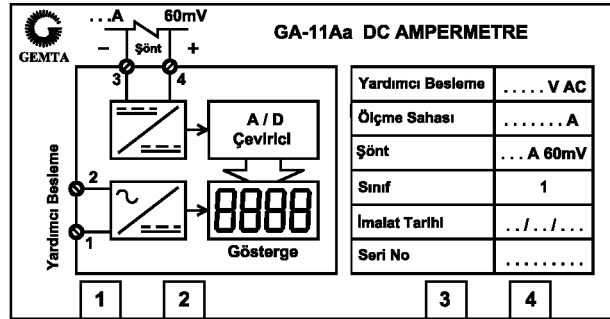
GA-11Aa BAĞLANTI ETİKETİ
