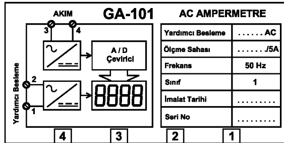
GA-101 BAĞLANTI ETİKETİ
